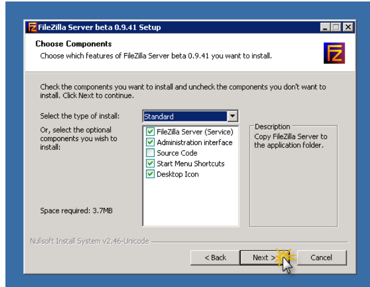
ภาพที่ ก.16 หน้าโปรแกรมติดตั้งของ FileZilla
